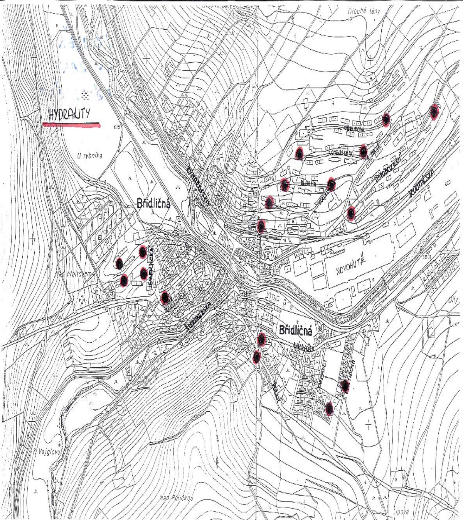
B) plánec obce s vyznačením zdrojů vody pro hašení požárů, čerpacích stanišť
